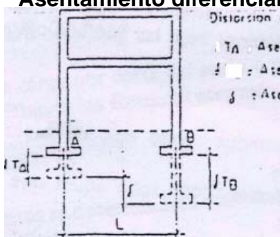
FIGURA N° 3 Asentamiento diferencial
