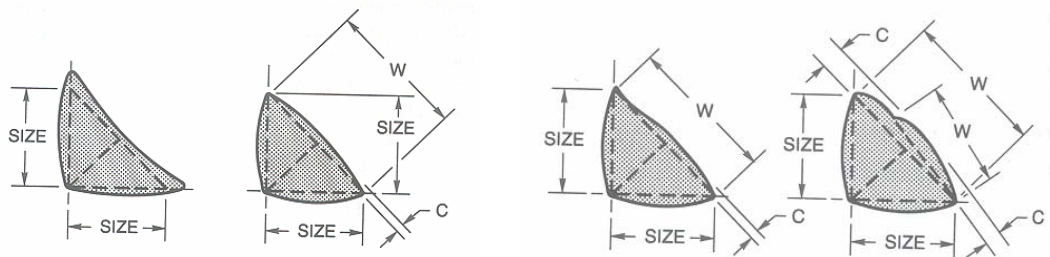
A) Perfiles de Soldadura de Filete Deseables
