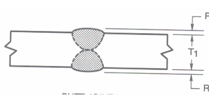
UNION A TOPE – PLANCHAS DE IGUAL ESPESOR
